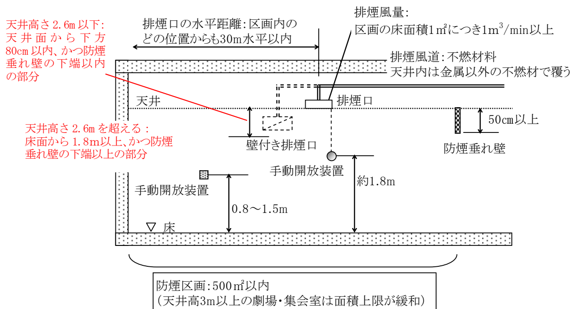
図 10.1 排煙設備の構造
